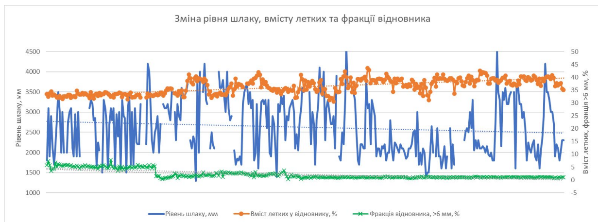
Малюнок 10. Зміна рівня шлаку, вмісту летких та фракції відновника.
