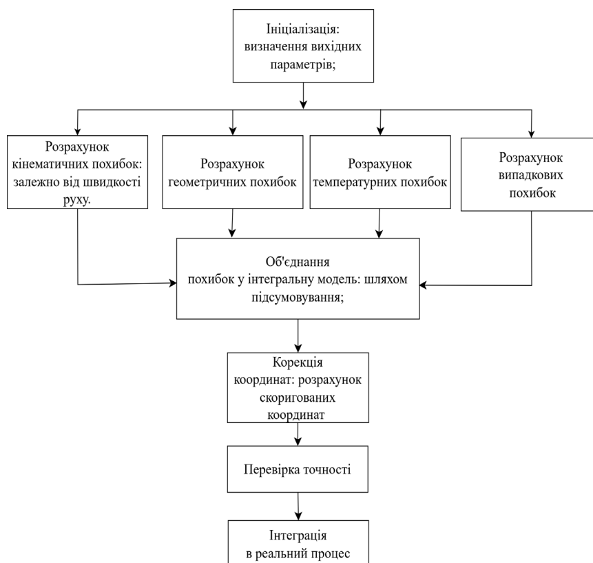
Рисунок 1. алгоритм корекції похибок на КВМ
